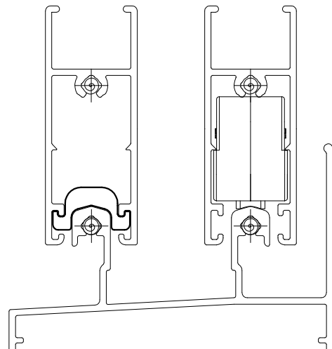
DETALHE DE UTILIZAÇÃO - ESC. 1-1
