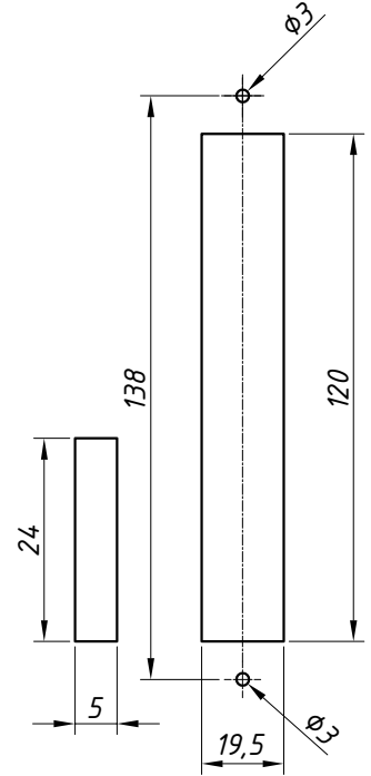
USINAGEM: (escala 1:2)
