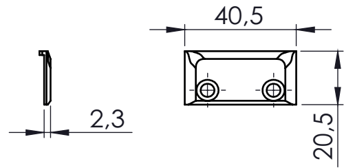
DIMENSÕES ESCALA 1:2
