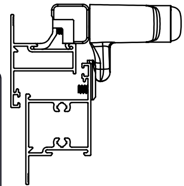
APLICAÇÃO ESCALA 1:2
