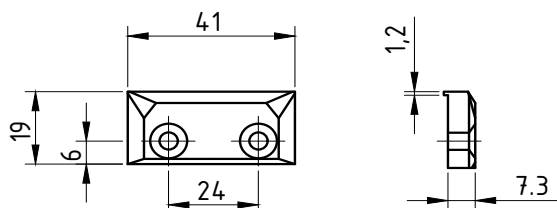
CONTRAFECHO: (escala 1:2)
