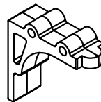
BATENTE SUPERIOR
