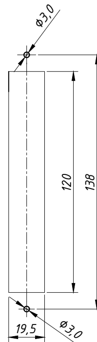
USINAGEM: (escala 1:2)
