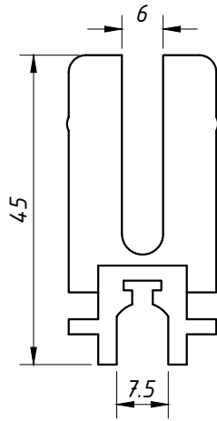
PESPECTIVA: (escala 1:1)
