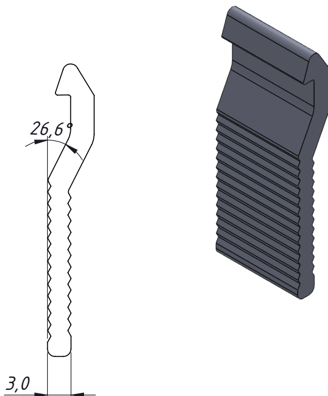
Perspectiva Escala 2:1
