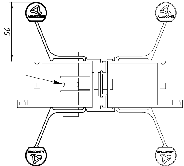
DETALHE DE APLICAÇÃO: (escala 1:2)
