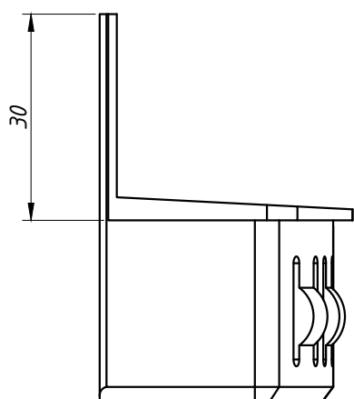
DIMENSÕES: (escala 1:1)
