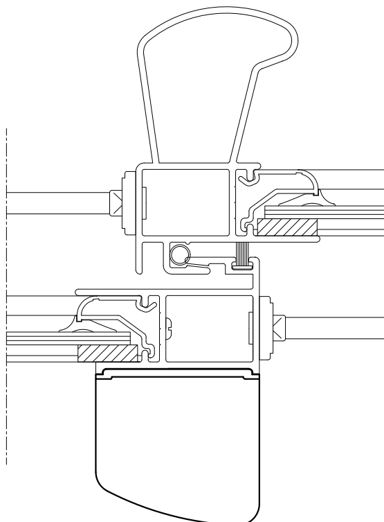
DETALHE DE APLICAÇÃO: (sem escala)
