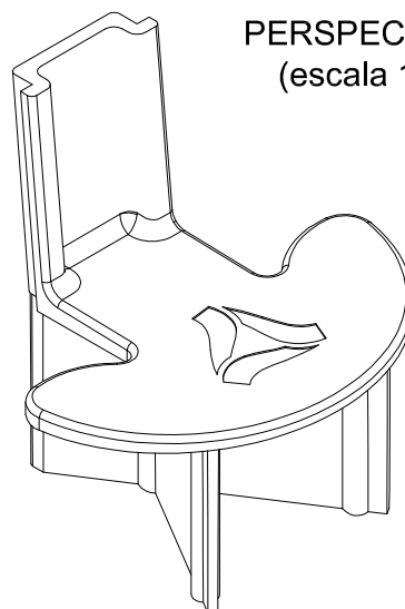
DETALHE DE APLICAÇÃO: (sem escala)
