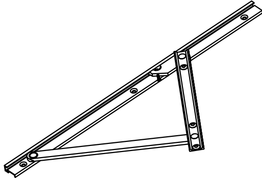
PERSPECTIVA: (sem escala)
