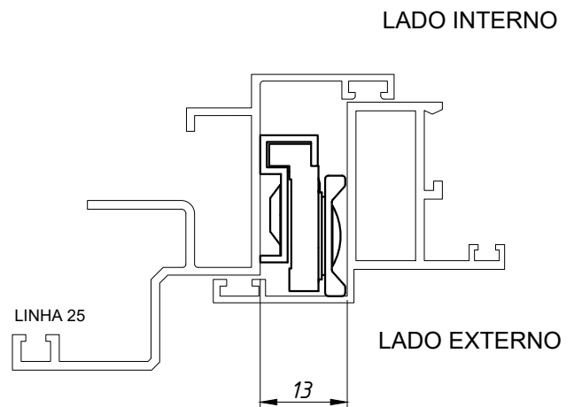
DETALHE DE APLICAÇÃO: (escala 1:1)
