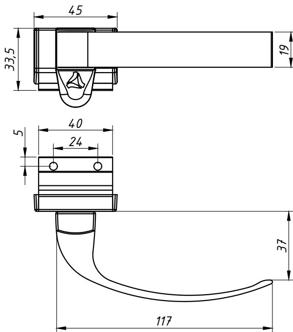
DIMENSÕES: (escala 1:2)
