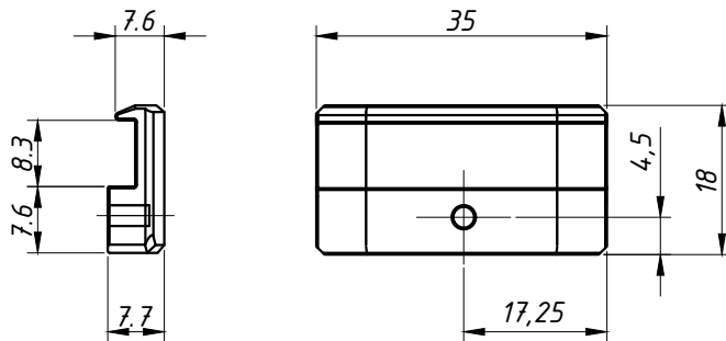
CONTRAFECHO: (escala 1:1)
