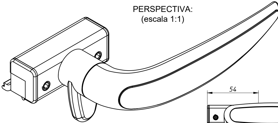
DIMENSÕES: (escala 1:2)
