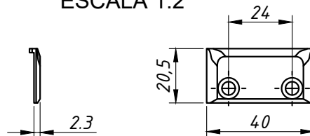
CONTRA FECHO: ESCALA 1:2
