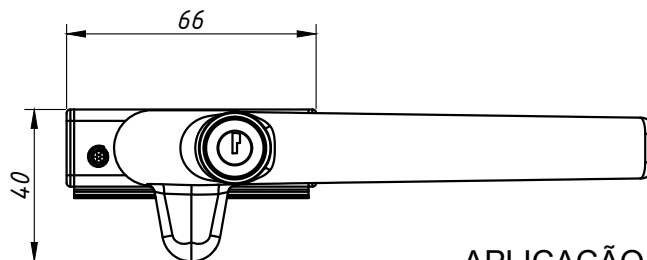
APLICAÇÃO ESCALA 1:2
