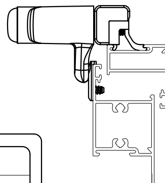
APLICAÇÃO ESCALA 1:2
