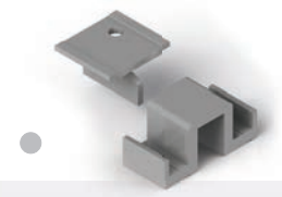
Contrafecho da Folha Fixa LINHAS: GOLD, MEGA 32, NOSTRA® 32, D'ORO e ALUK 3.2 CÓD.: CON-32
