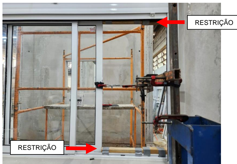
Figura 3 – Instrumentação de ensaio de resistência horizontal com dois cantos imobilizados
