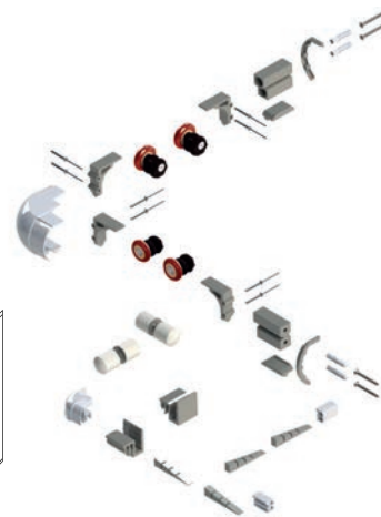
Kit Box 4 CÓD.: KIT-04 CORES: Preto, Branco, Cinza, Cromado, Bronze 1002, Bronze 1001
