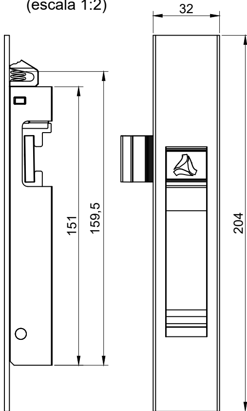
DIMENSÕES: (escala 1:2)
