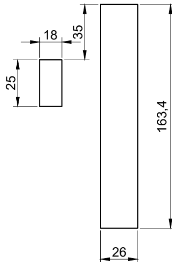
USINAGEM: (escala 1:2)
