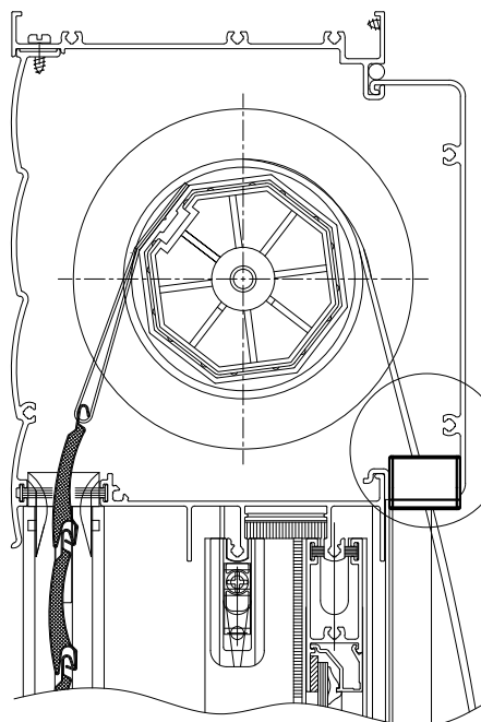
Detalhe de Montagem (S/ Escala)
