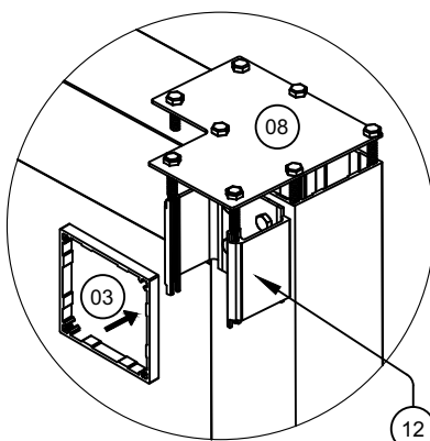
DETALHE E-E
