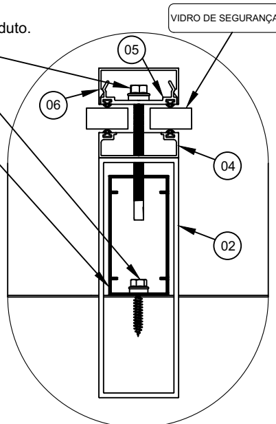
DETALHE F-F
