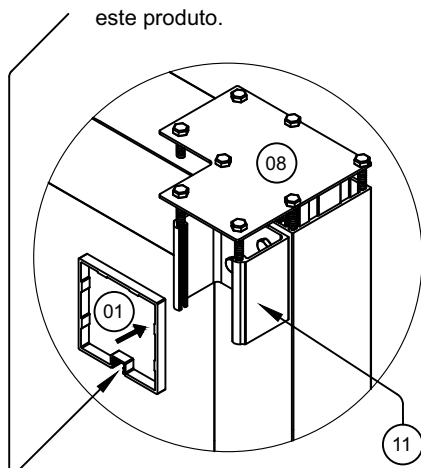
DETALHE D-D
