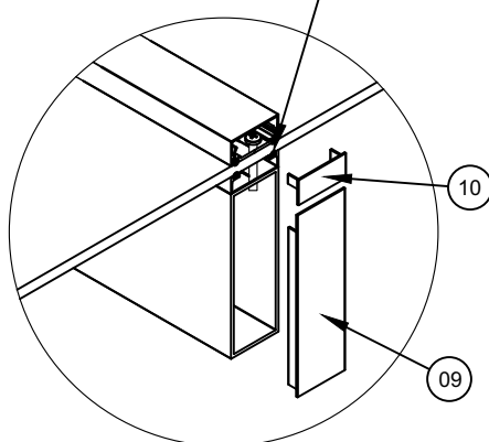
DETALHE A-A
