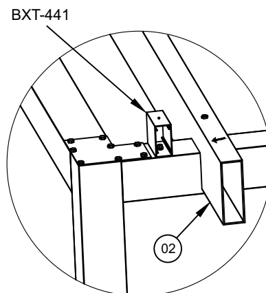
DETALHE C-C
