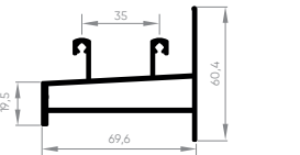
EXL-006 Trilho intermediário inferior 1,145 Kg/m
