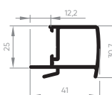
EXL-501 Montante central interno da folha 0,479 Kg/m
