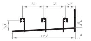
ALV-2006 Matajunta lateral 0,382 Kg/m
