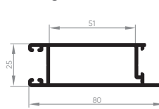
ALV-2082 Montante lateral da folha 0,803 Kg/m
