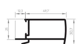
ALV-2018 Montante central interno da folha 0,626 Kg/m
