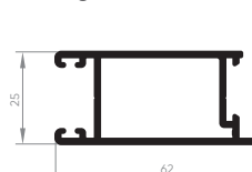
ALV-2017 Montante lateral da folha 0,653 Kg/m
