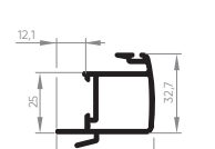
EXL-503 Montante central intermediário da folha 0,549 Kg/m
