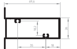
EXL-009 Travessa 70 mm 0,908 Kg/m
