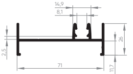
EXL-791 Marco lateral de correr 2 planos com contrafecho 0,559 Kg/m
