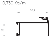
ALV-2027 Montante intermediário da folha 60 0,730 Kg/m
