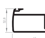
ALV-2015 Montante central externo da folha 0,690 Kg/m
