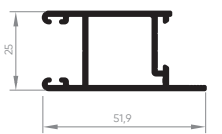
EXL-500 Montante lateral da folha 0,528 Kg/m
