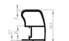
EXL-400 Montante bi-tubular central interno reforçado 1,038 Kg/m
