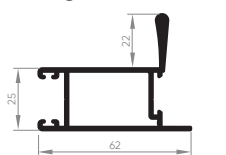
ALV-2014 Montante central da folha 0,842 Kg/m
