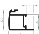
EXL-502 Montante central externo da folha 0,512 Kg/m
