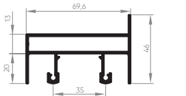
EXL-005 Trilho intermediário superior 1,107 Kg/m
