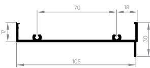
EXL-018 Perfil travessa bandeira 03 planos 0,670 kg/m
