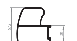
ALV-2016 Montante bi-tubular central interno da folha 0,911 Kg/m
