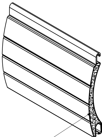
PERSPECTIVA: (escala 1:1)
