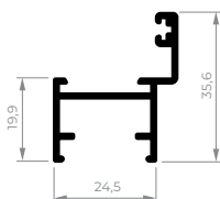
CEL-079 Travessa da folha 0,338 kg/m
