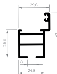
CEL-200 Montante maxim-ar com escova 0,478 kg/m
