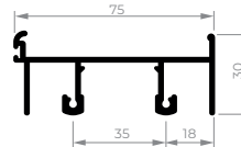
CEL-509 Marco intermediário integrada 0,784 kg/m
