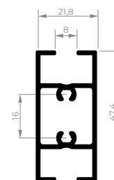
CEL-227 Travessa intermediária da folha | 0,600 kg/m
