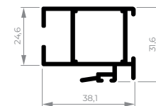
CEL-245 Montante lateral da folha 0,668 kg/m
