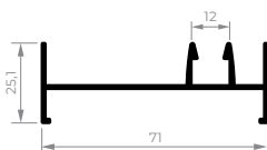
CEL-791 Marco lateral com contrafecho 0,500 kg/m
