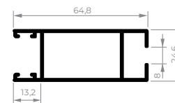
CEL-245 Montante lateral da folha 0,668 kg/m
