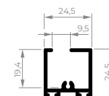
CEL-193 Montante marco basculante 0,329 kg/m
