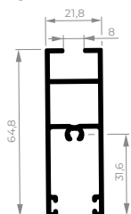
CEL-246 Travessa inferior da folha 0,686 kg/m
