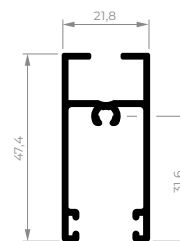
CEL-053 Travessa da folha 0,473 kg/m
