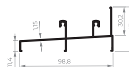
CEL-510 Trilho inferior integrada 0,775 kg/m
