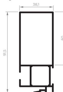
CEL-060 Montante central da folha com reforço 1,026 kg/m
