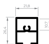
CEL-082 Travessa inferior maxim-ar 0,380 kg/m
