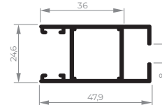
CEL-039 Montante da folha 0,545 kg/m
