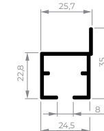
CEL-194 Travessa marco basculante 0,321 kg/m
