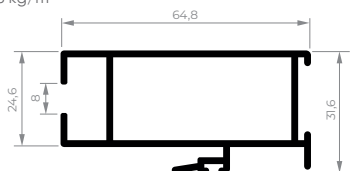
CEL-243 Montante central interno 0,735 kg/m
