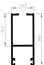
CEL-514 Guia para persiana 0,519 kg/m
