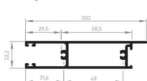
EXL-225 Travessa inferior porta 0,892 Kg/m
