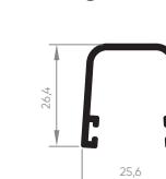
EXL-107 Vedação do montante 0,272 Kg/m
