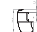
EXL-505 Montante bitubular central externo 0,803 Kg/m
