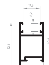
EXL-039 Montante da folha 0,551 Kg/m
