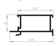
EXL-243 Montante central interno 0,668 Kg/m
