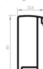
ALV-2081 Montante central externo da folha 0,834 Kg/m
