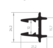
EXL-506 Mata-junta central da folha 0,303 Kg/m
