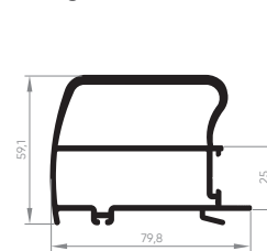
ALV-2088 Montante bitubular central interno da folha 80 1,617 Kg/m
