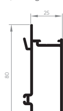
ALV-2080 Montante central interno da folha 0,854 Kg/m
