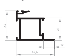
EXL-041 Montante central externo 0,505 Kg/m
