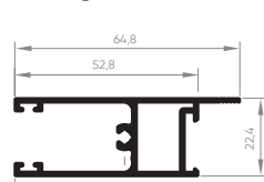
EXL-246 Travessa inferior da folha 0,645 Kg/m
