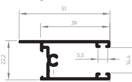
EXL-053 Travessa da folha 0,447 Kg/m
