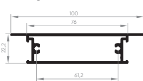
EXL-050 Travessa intermediária da folha 0,924 Kg/m
