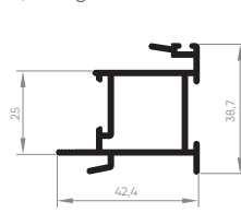
EXL-042 Montante central intermediário 0,556 Kg/m
