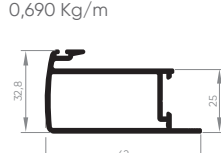
ALV-2015 Montante central externo da folha 0,690 Kg/m
