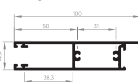
EXL-666 Travessa inferior porta 0,974 Kg/m
