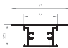
EXL-227 Travessa intermediária da folha 0,556 Kg/m
