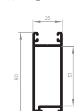
ALV-2082 Montante lateral da folha 0,801 Kg/m
