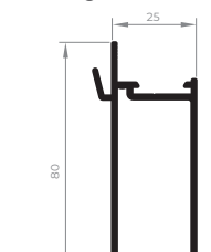
ALV-2084 Montante intermediário da folha 80 0,872 Kg/m
