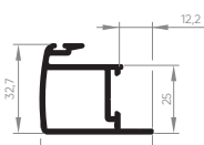
EXL-502 Montante central externo da folha 0,512 Kg/m
