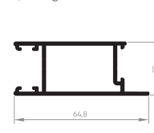
EXL-245 Montante lateral da folha 0,623 Kg/m
