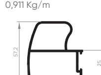
ALV-2016 Montante bitubular central interno da folha 0,911 Kg/m
