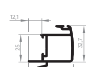
EXL-503 Montante central intermediário da folha 0,549 Kg/m
