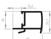
EXL-501 Montante central interno da folha 0,479 Kg/m
