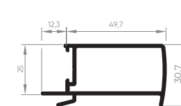
ALV-2018 Montante central interno da folha 0,626 Kg/m
