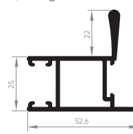
EXL-250 Montante central da folha 0,796 Kg/m
