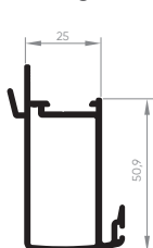
ALV-2027 Montante intermediário da folha 60 0,730 Kg/m
