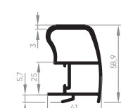
EXL-400 Montante bitubular central interno reforçado 1,038 Kg/m
