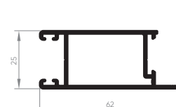
ALV-2017 Montante lateral da folha 0,653 Kg/m
