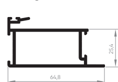
EXL-242 Montante central externo 0,743 Kg/m
