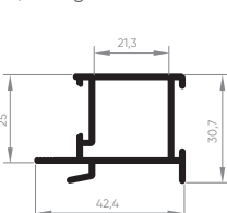
EXL-040 Montante central interno 0,474 Kg/m
