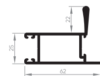
ALV-2014 Montante central da folha 0,842 Kg/m
