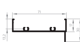
EXL-004 Marco superior e inferior 0,485 Kg/m
