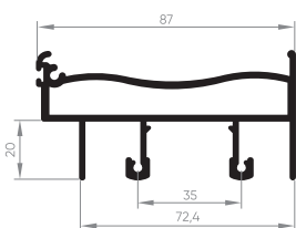
EXL-507 Marco intermediário integrada tubular 1,331 Kg/m
