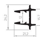
EXL-506 Matajunta central da folha 0,303 Kg/m
