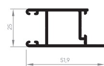
EXL-500 Montante lateral da folha 0,528 Kg/m
