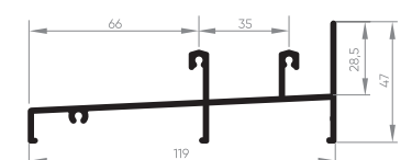
EXL-510 Trilho inferior integrada 1,062 Kg/m
