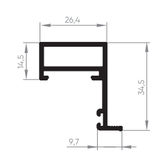
AFV-008 Folha colada 0,396 Kg/m
