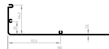
EXL-032 Tampa interna janela integrada 1,494 Kg/m
