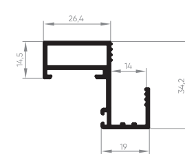
AFV-007 Folha encaixilhada 0,542 Kg/m
