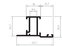
EXL-200 Montante com escova maxim-ar 0,419 Kg/m
