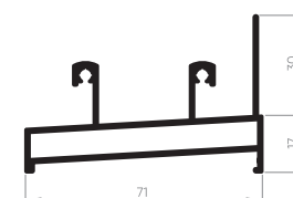
EXL-998 Trilho de correr inferior 2 planos 0,923 Kg/m
