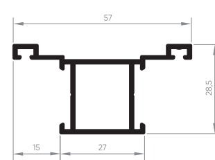
EXL-085 Travessa vertical sem alhal maxim-ar 0,491 Kg/m
