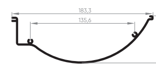
EXL-517 Tampa interna porta integrada 1,074 Kg/m
