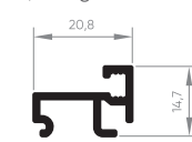
ALV-2042 Baguete mosquiteira travessa 0,195 Kg/m
