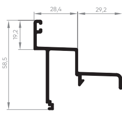
AFV-006 Batente inferior 0,676 Kg/m
