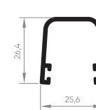
EXL-107 Vedação do montante 0,272 Kg/m
