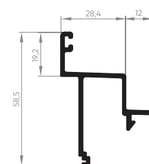
AFV-012 Batente inferior sem pingadeira 0,577 Kg/m
