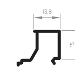
EXL-103 Baguete para Marco 0,126 Kg/m
