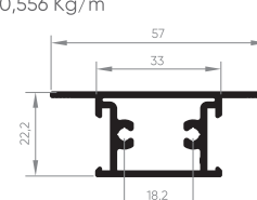
EXL-506 Matajunta central da folha 0,303 Kg/m
