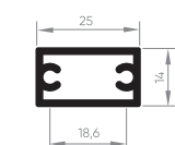
ALV-2706 Tubo retangular com alhal 0,313 Kg/m
