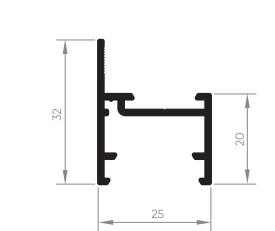
EXL-088 Marco perimetral fixo 0,278 Kg/m
