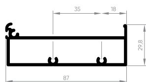
AFV-004 Marco intermediário tubular liso 1,085 Kg/m
