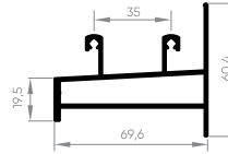
EXL-006 Trilho intermediário inferior 1,145 Kg/m
