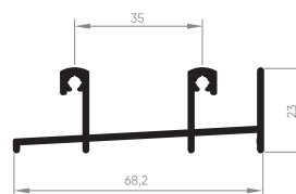
EXL-260 Trilho de correr inferior porta 2 planos 0,555 Kg/m
