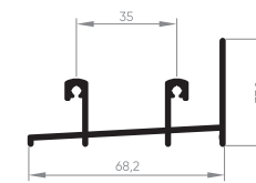
EXL-228 Trilho de correr inferior 2 planos 0,600 Kg/m
