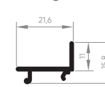
ALV-2044 Baguete Vidro Duplo/Veneziana 0,139 Kg/m
