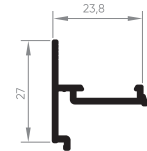
AFV-006 Batente inferior 0,676 Kg/m
