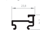
ALV-2043 Baguete mosquiteira montante 0,190 Kg/m
