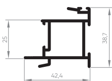
EXL-1502 Perfil montante central ext. Folha 0,593 Kg/m
