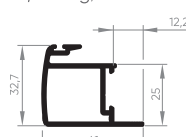
EXL-502 Montante central externo da folha 0,540 Kg/m
