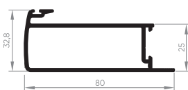
EXL-042 Montante central intermediário 0,556 Kg/m
