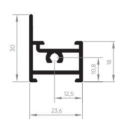
EXL-082 Travessa superior maxim-ar 90° 0,382 Kg/m
