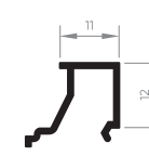
EXL-102 Baguete 0,102 Kg/m
