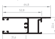
EXL-246 Travessa inferior da folha 0,645 Kg/m
