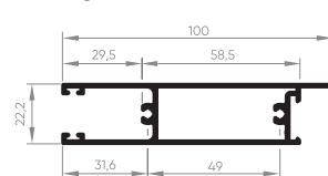
EXL-225 Travessa inferior porta 0,892 Kg/m
