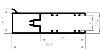
EXL-800 Perfil trilho persiana 55 mm 0,972 Kg/m
