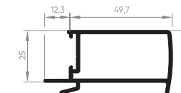
ALV-2018 Montante central interno da folha 0,626 Kg/m
