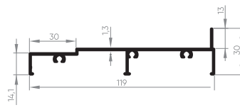
EXL-802 Marco inferior integrada c/ peitoril 0,757 Kg/m
