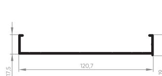
EXL-511 Marco lateral integrada 0,578 Kg/m
