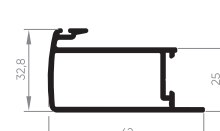
ALV-2015 Montante central externo da folha 0,690 Kg/m
