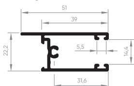
EXL-053 Travessa da folha 0,447 Kg/m
