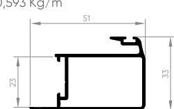
EXL-1502 Perfil montante central ext. Folha 0,593 Kg/m
