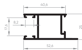
EXL-039 Montante da folha 0,551 Kg/m
