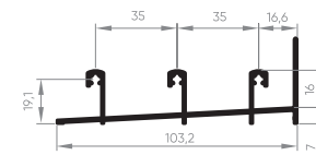
ALV-2042 Baguete mosquiteira travessa 0,195 Kg/m
