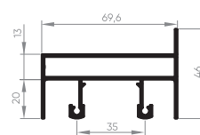
EXL-005 Trilho intermediário superior 1,107 Kg/m
