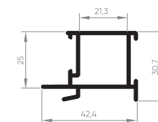
EXL-242 Montante central externo 0,743 Kg/m
