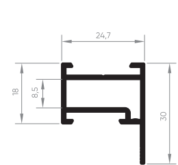
EXL-080 Travessa superior maxim-ar 45° 0,320 Kg/m
