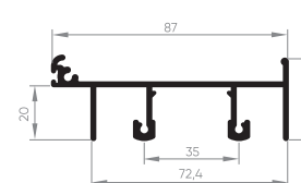
EXL-509 Marco intermediário integrada 0,802 Kg/m
