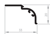
EXL-276 Pingadeira do marco maxim-ar 0,176 Kg/m
