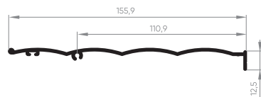
EXL-516 Tampa externa janela integrada 0,698 Kg/m
