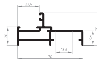
ALV-2708 Marco com suporte grade 0,711 Kg/m
