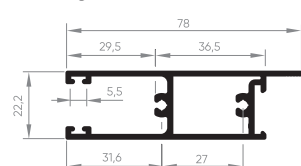
EXL-224 Travessa inferior da folha 0,790 Kg/m
