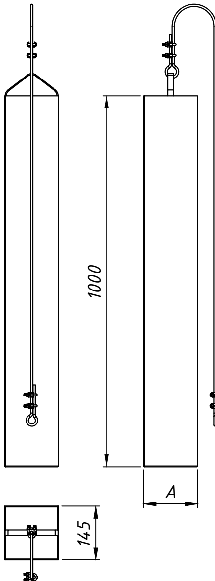
DIMENSÕES: (Escala 1:10)
