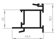
EXL-042 Montante central intermediário 0,556 Kg/m
