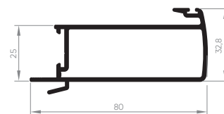
EXL-245 Montante lateral da folha 0,641 Kg/m
