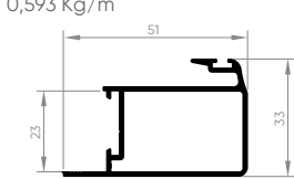
EXL-1502 Perfil montante central ext. Folha 0,593 Kg/m
