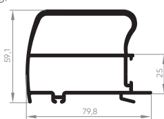
EXL-250 Montante central da folha 0,796 Kg/m
