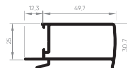
ALV-2018 Montante central interno da folha 0,626 Kg/m
