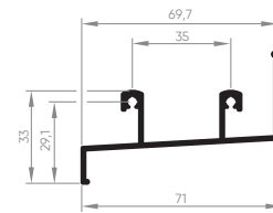
EXL-002 Trilho de correr inferior 2 planos 0,686 Kg/m
