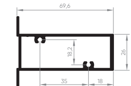
EXL-009 Travessa 70 mm 0,908 Kg/m
