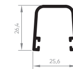
EXL-107 Vedação do montante 0,272 Kg/m
