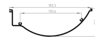
EXL-517 Tampa interna porta integrada 1,074 Kg/m
