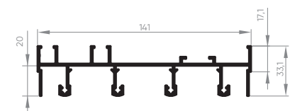
EXL-121 Trilho de correr superior 4 planos 1,577 Kg/m
