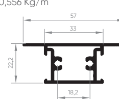
EXL-506 Matajunta central da folha 0,303 Kg/m
