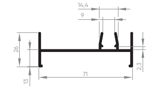
EXL-003 Marco lateral de correr 2 planos 0,517 Kg/m
