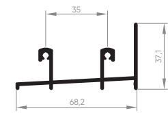
EXL-228 Trilho de correr inferior 2 planos 0,600 Kg/m
