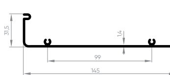
EXL-031 Tampa interna janela integrada 0,941 Kg/m
