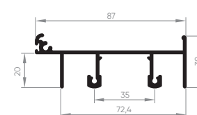
EXL-509 Marco intermediário integrada 0,802 Kg/m
