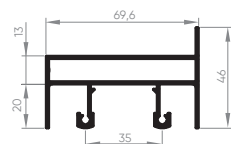
EXL-005 Trilho intermediário superior 1,107 Kg/m
