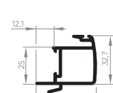
EXL-503 Montante central intermediário da folha 0,549 Kg/m
