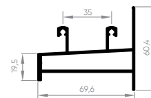
EXL-006 Trilho intermediário inferior 1,145 Kg/m
