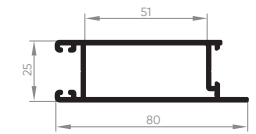
ALV-2082 Montante lateral da folha 0,803 Kg/m
