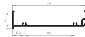
EXL-508 Marco superior integrada 0,794 Kg/m
