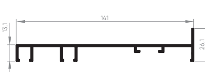
EXL-123 Montante lateral de correr 4 planos 0,871 Kg/m
