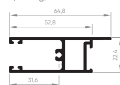
EXL-246 Travessa inferior da folha 0,645 Kg/m
