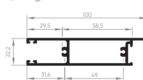
EXL-225 Travessa inferior porta 0,923 Kg/m
