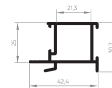
EXL-242 Montante central externo 0,743 Kg/m
