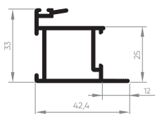
EXL-041 Montante central externo 0,505 Kg/m
