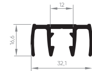
ALV-2006 Matajunta lateral 0,382 Kg/m
