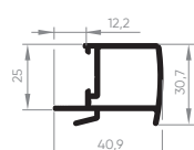
EXL-501 Montante central interno da folha 0,479 Kg/m
