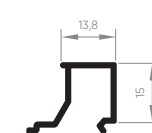
EXL-103 Baguete para Marco 0,126 Kg/m
