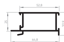
EXL-243 Montante central interno 0,668 Kg/m
