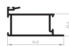
EXL-242 Montante central externo 0,743 Kg/m
