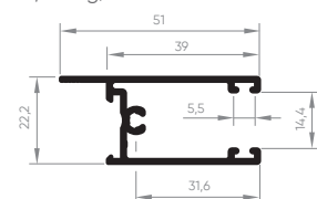
EXL-053 Travessa da folha 0,481 Kg/m
