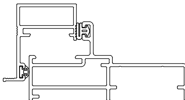
BT001 - VEDAÇÃO DA FOLHA
