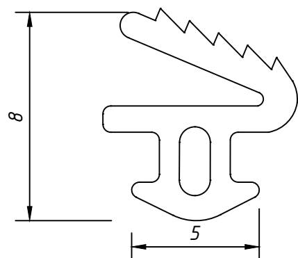
BT002 - VEDAÇÃO DO MARCO
