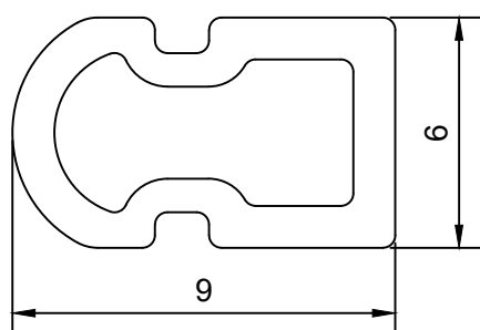
BT007 - VEDAÇÃO DO MONTANTE CENTRAL NOSTRA 32 SEM BAGUETE
