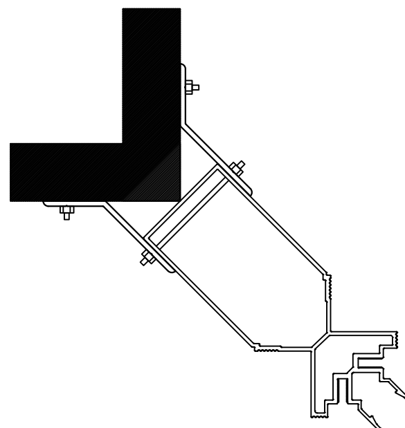
DETALHE DE APLICAÇÃO: (sem escala)
