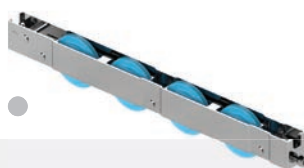
Forza 400 | Trilho "U" Roldana Quádrupla com Rolamento e Regulagem para Escova Inferior
