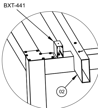
DETALHE C-C
