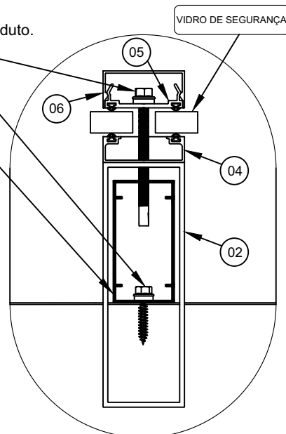
DETALHE F-F
