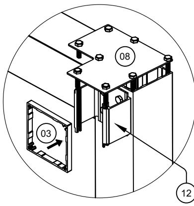
DETALHE E-E
