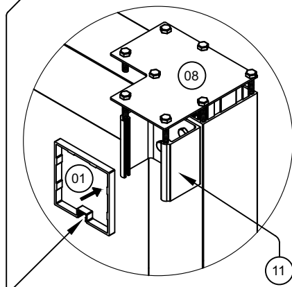
DETALHE D-D
