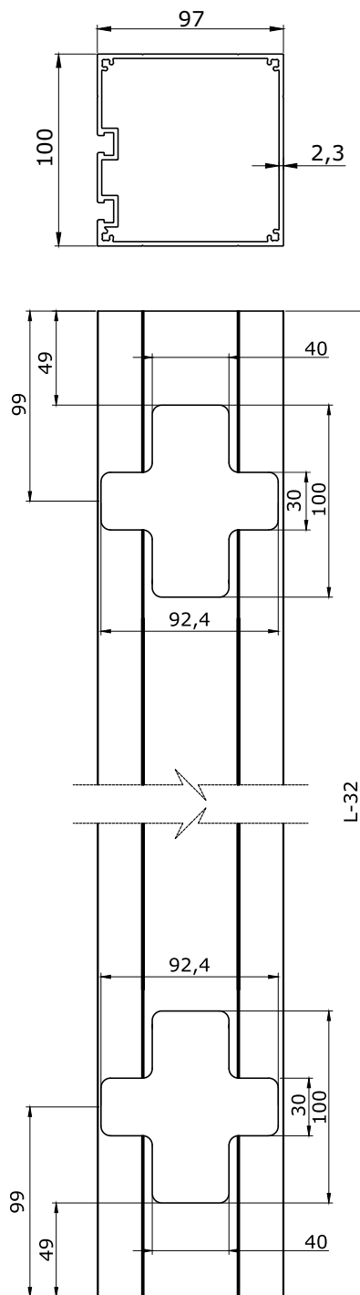
VISTA INFERIOR
